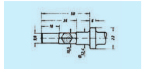
Abmessung Meißelschaft
