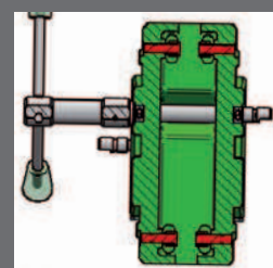
auf acht Stahlrollen gel. Schlitten (PLB 450), alle Stellelemente mit 19er Schlüsselweite
